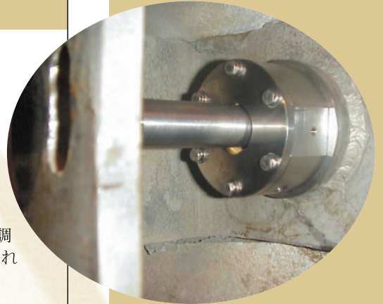
写真上： ロータリーバルブの シャフトに取り付けられた AHUシリーズシール
