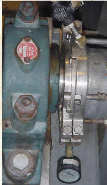
写真左： スパイス加工プロセスの リボンブレンダーに取り付 けられたAHS（分割型）
